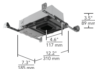
IC AIRTIGHT/CHICAGO PLENUM
